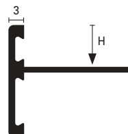
Sezione Alluminio
